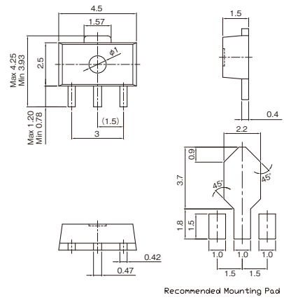
SOT 89 5
